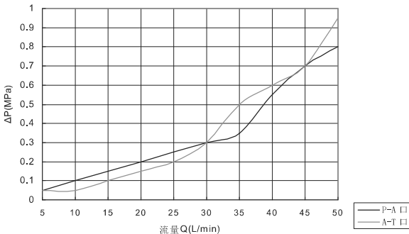
流量-压力损失曲线
